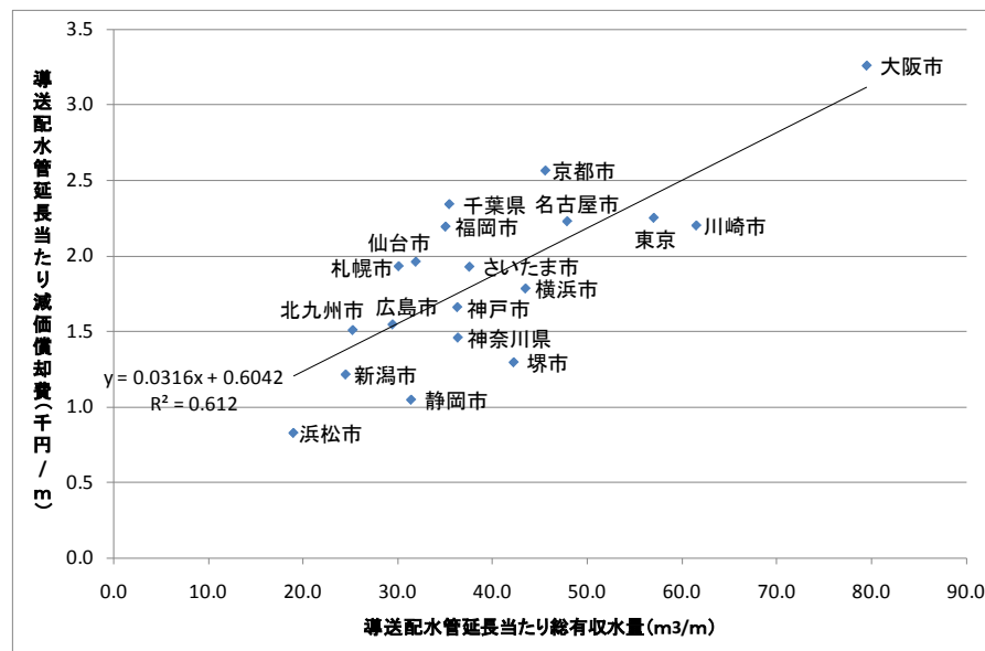
施設効率と減価償却費
