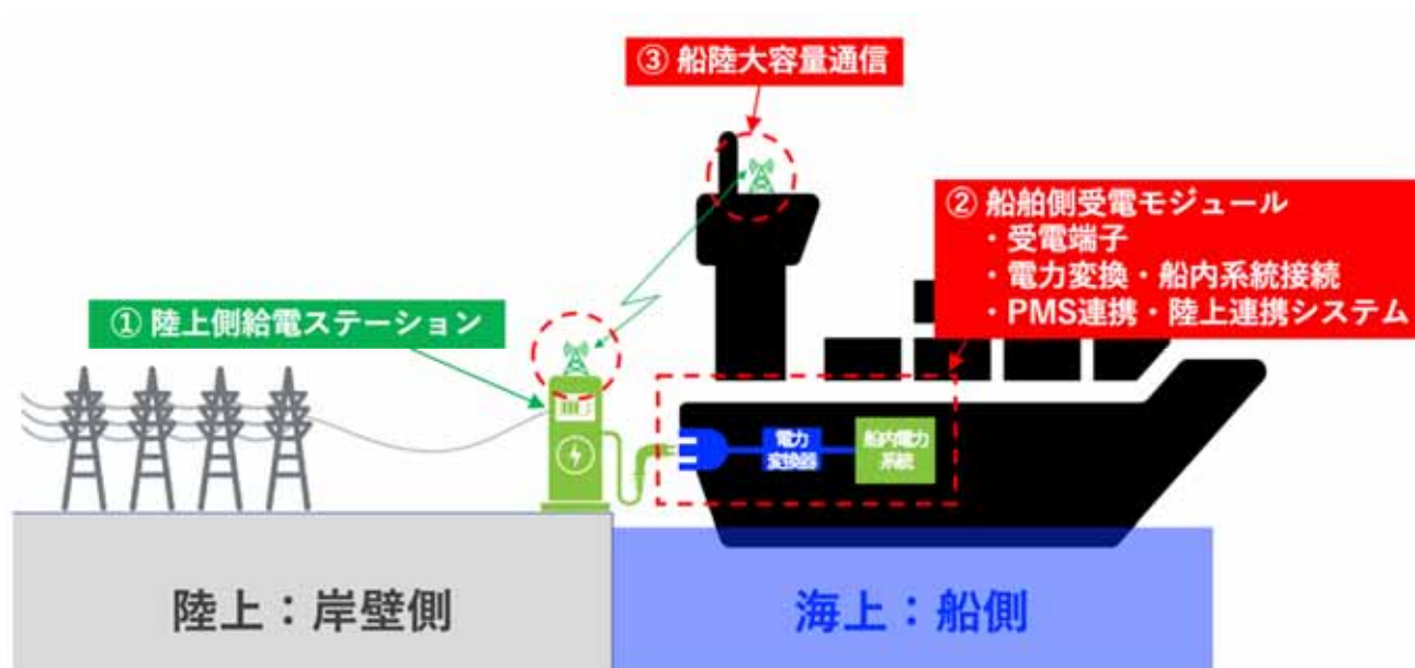
図1：船舶向け標準汎用型ゼロエミチャージャーシステムの構成イメージ
